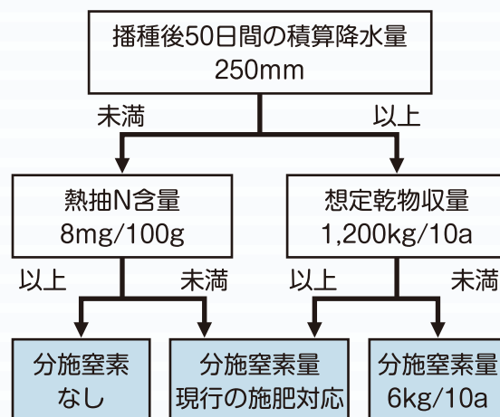
図2) 播種後の気象および窒素肥沃度に基づく分施窒素の施用方法
