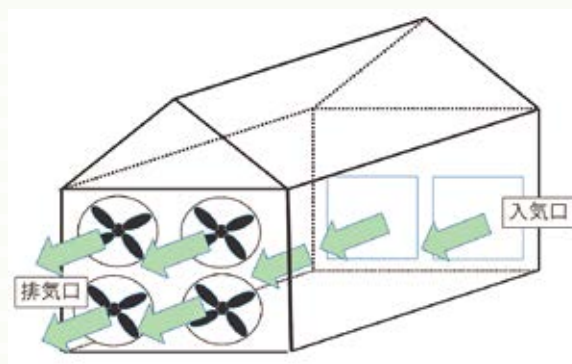
図3) トンネル換気の空気の流れ
