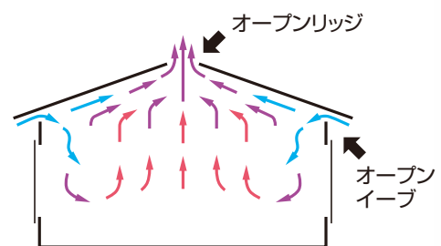
図2 気温差を利用した換気（冬季）
